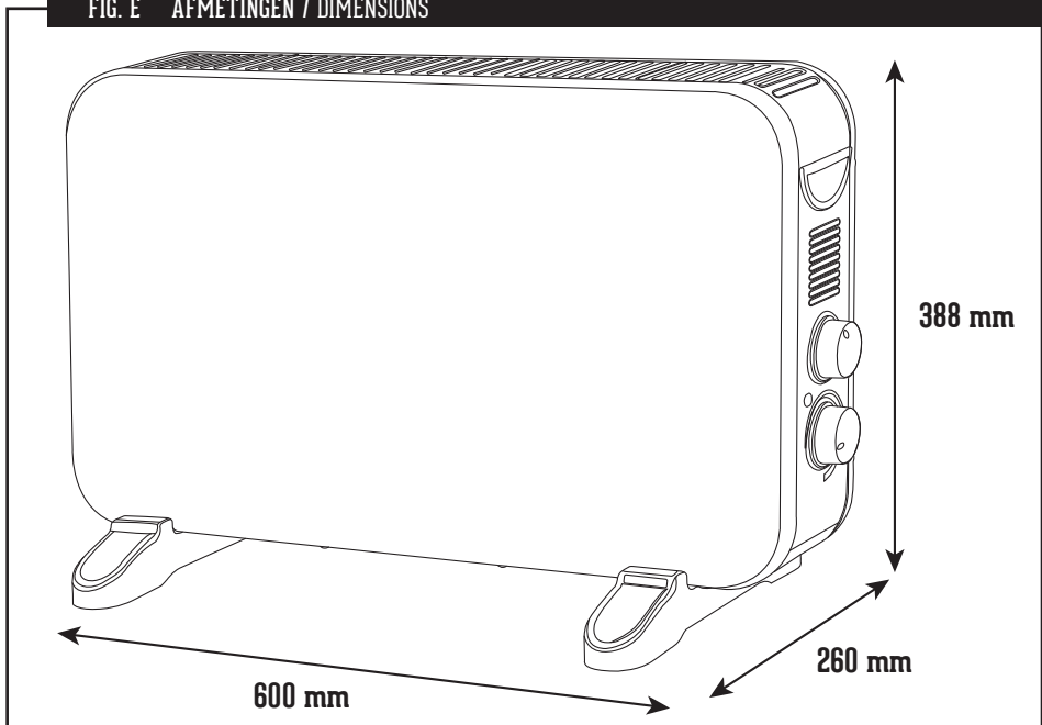
FIG. E AFMETINGEN / DIMENSIONS
